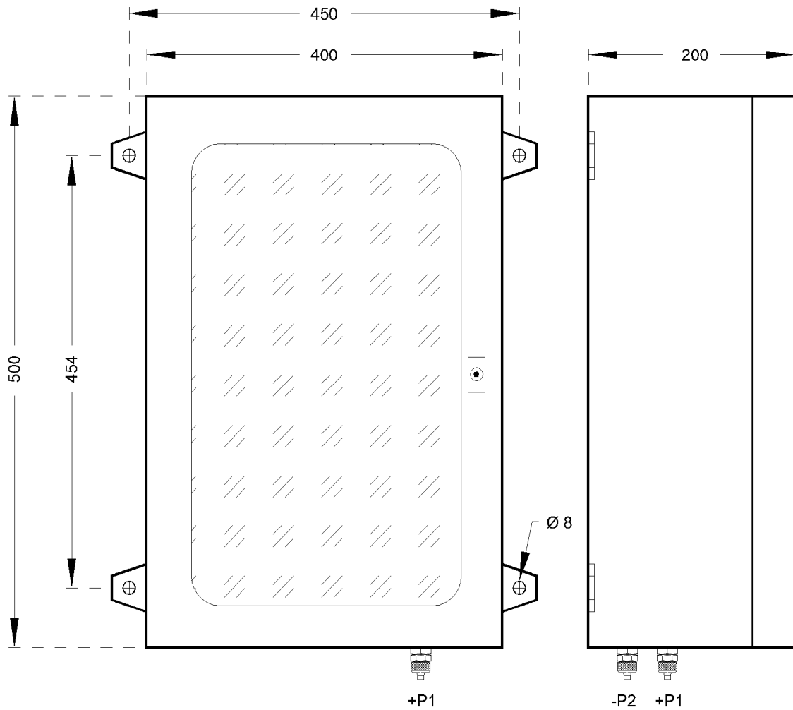
ABMESSUNGEN mm.
