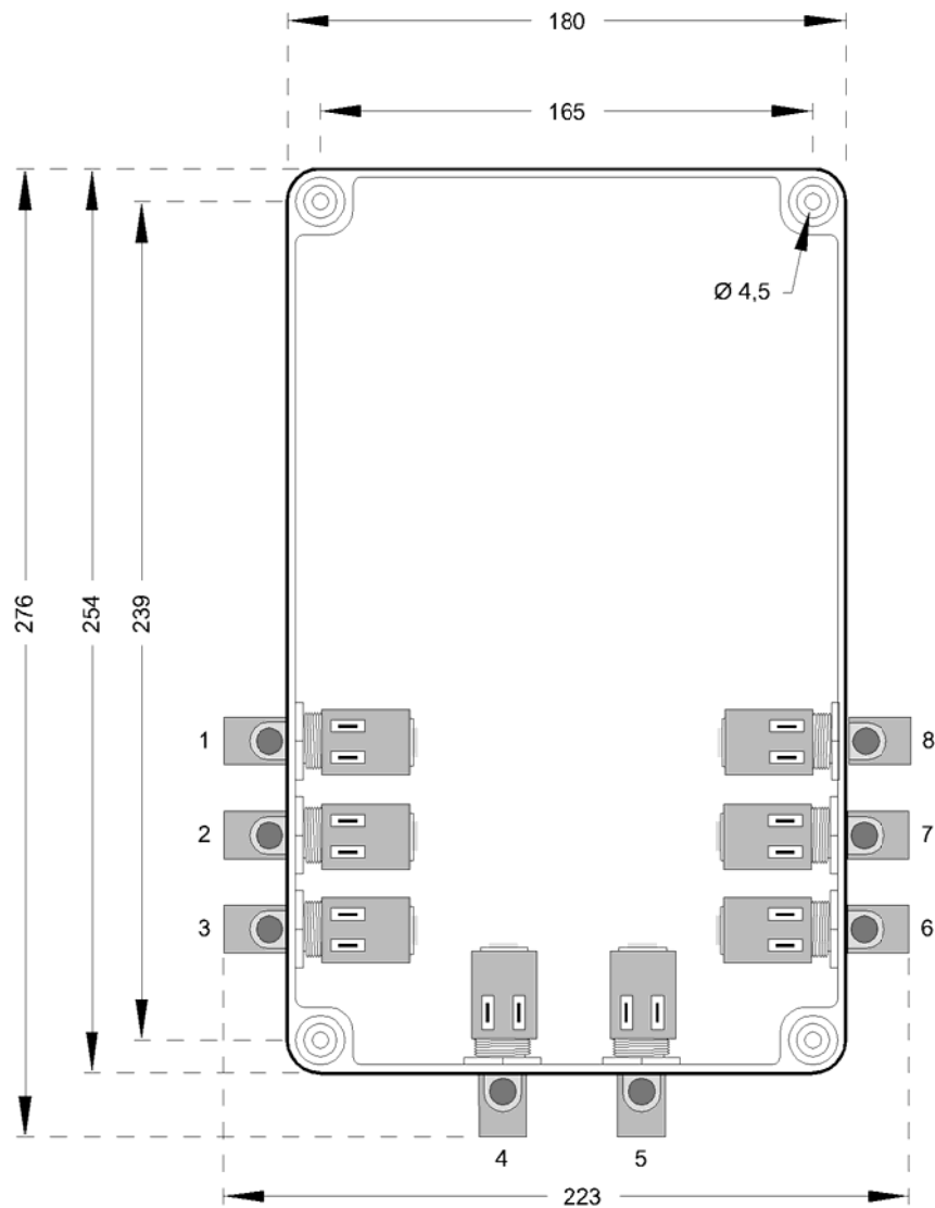
ABMESSUNGEN mm.
