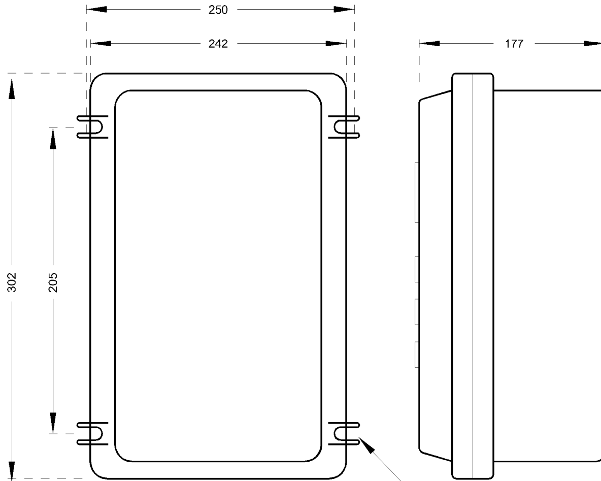
ABMESSUNGEN mm.
