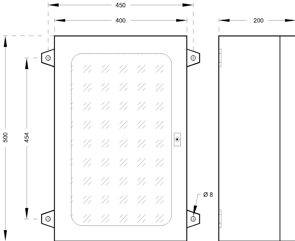
ABMESSUNGEN mm.
